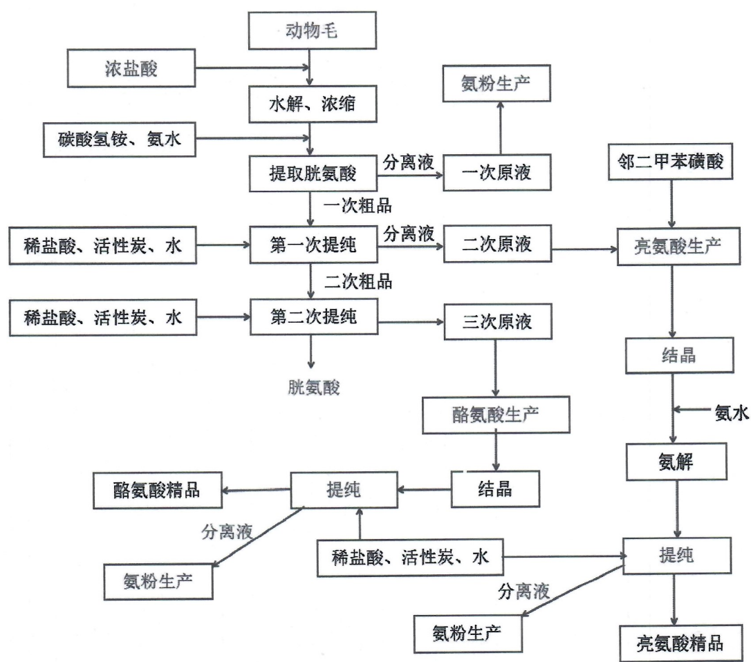
图 3.1-1 氨基酸提取工艺物料走向链图
