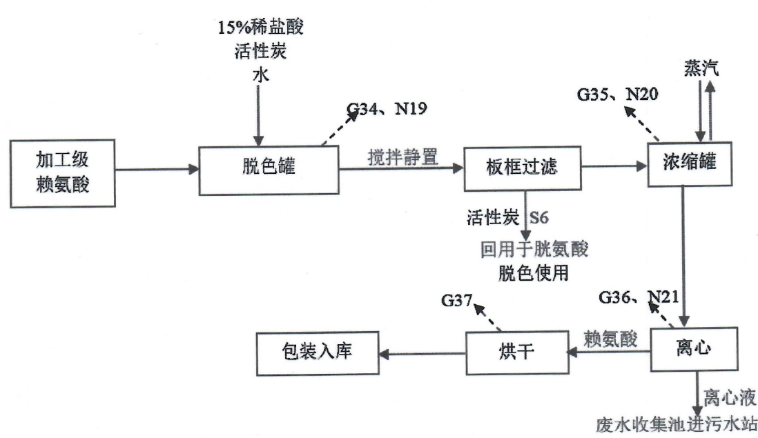
图 3.1-3 赖氨酸生产工艺流程简图
